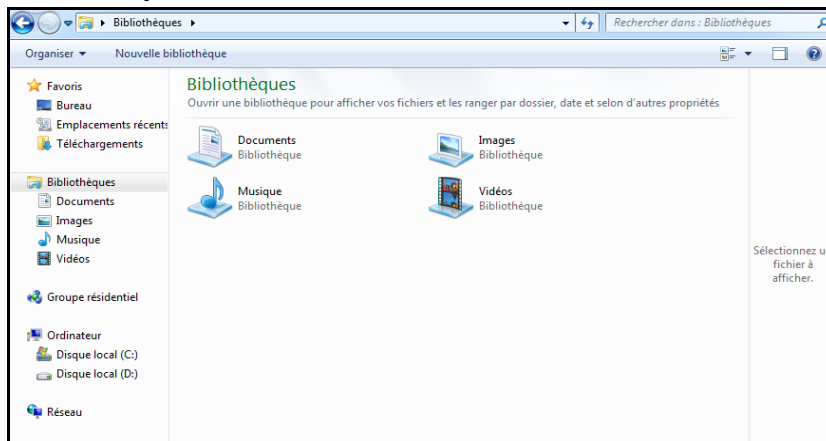
Explorateur Windows
